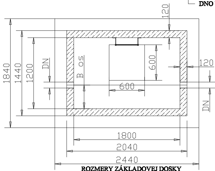
PÔDORYS
