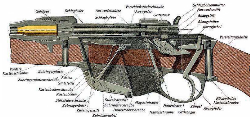
Mannlicher M1895.
