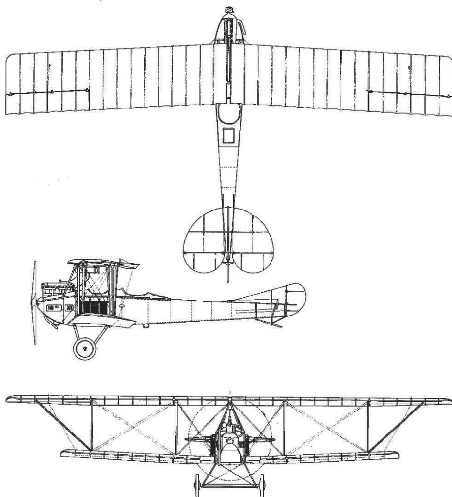
Aviatik B.I.
